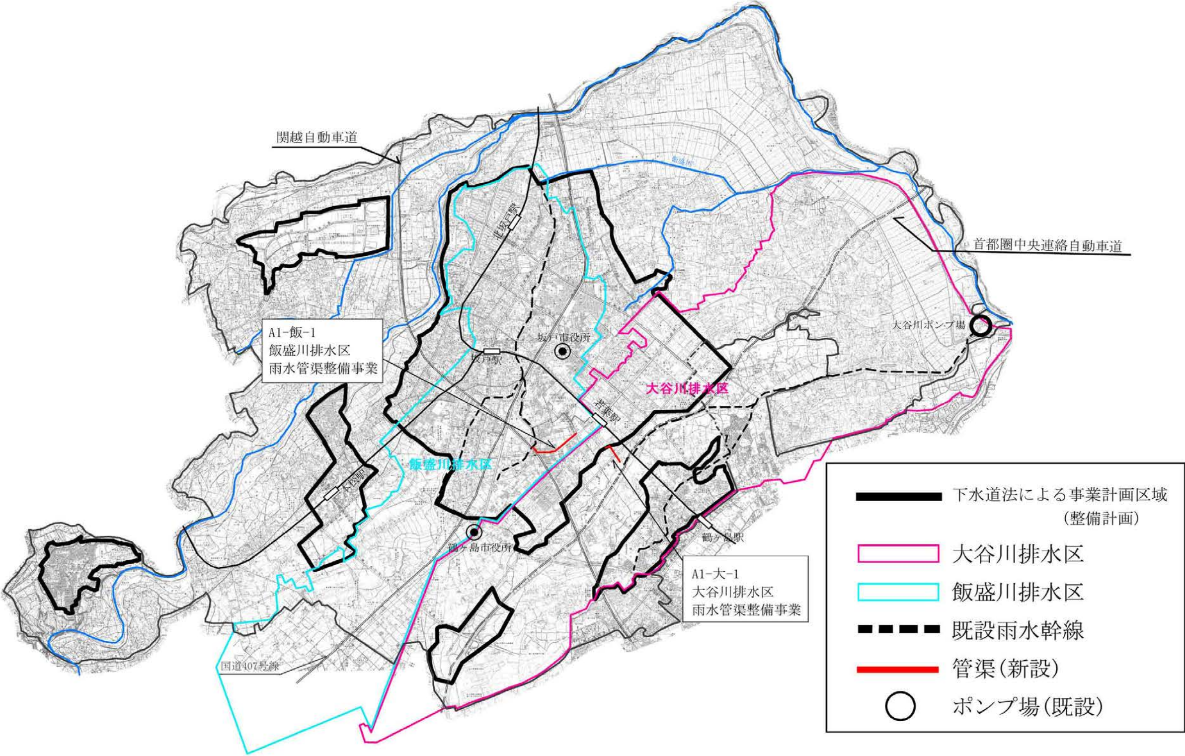
坂戸、鶴ヶ島下水道組合雨水計画図
